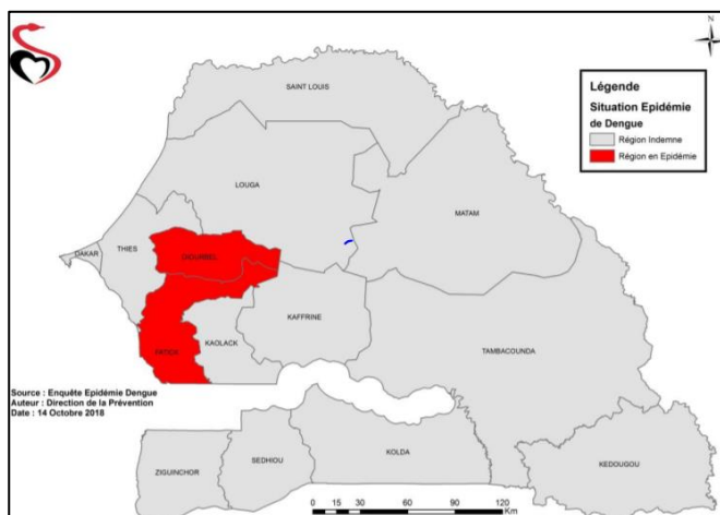
Fig. 1 : Localisation de l'épidémie de Dengue au Sénégal au 14 octobre 2018 / Location of the Dengue epidemic in Senegal as at 14 October 2018.
